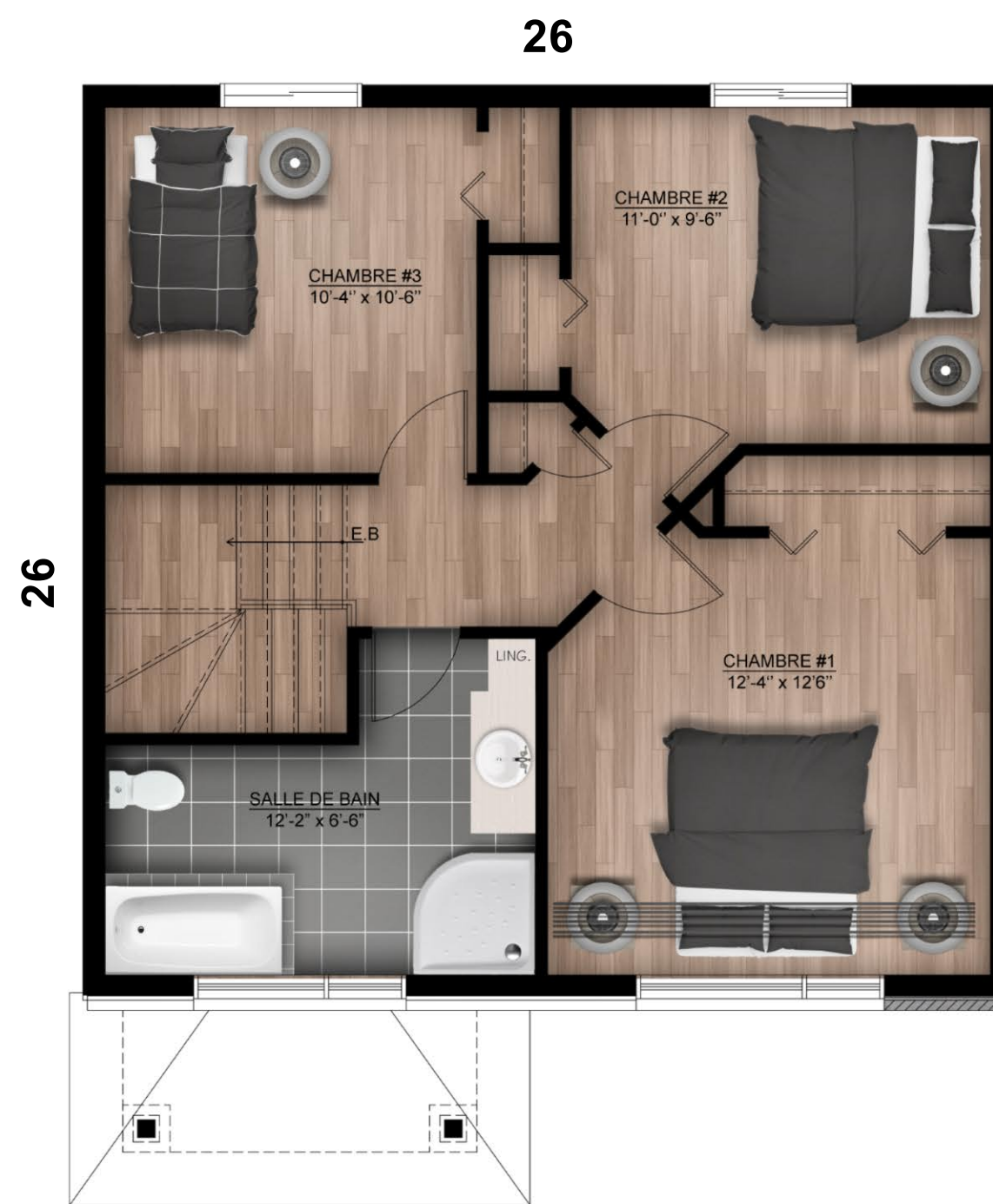
ÉTAGE SUP.TOTALE: +/- 676 pi.ca. MONACO 5
